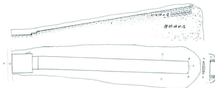
图1-2 衡州窑——龙窑平、剖面图
